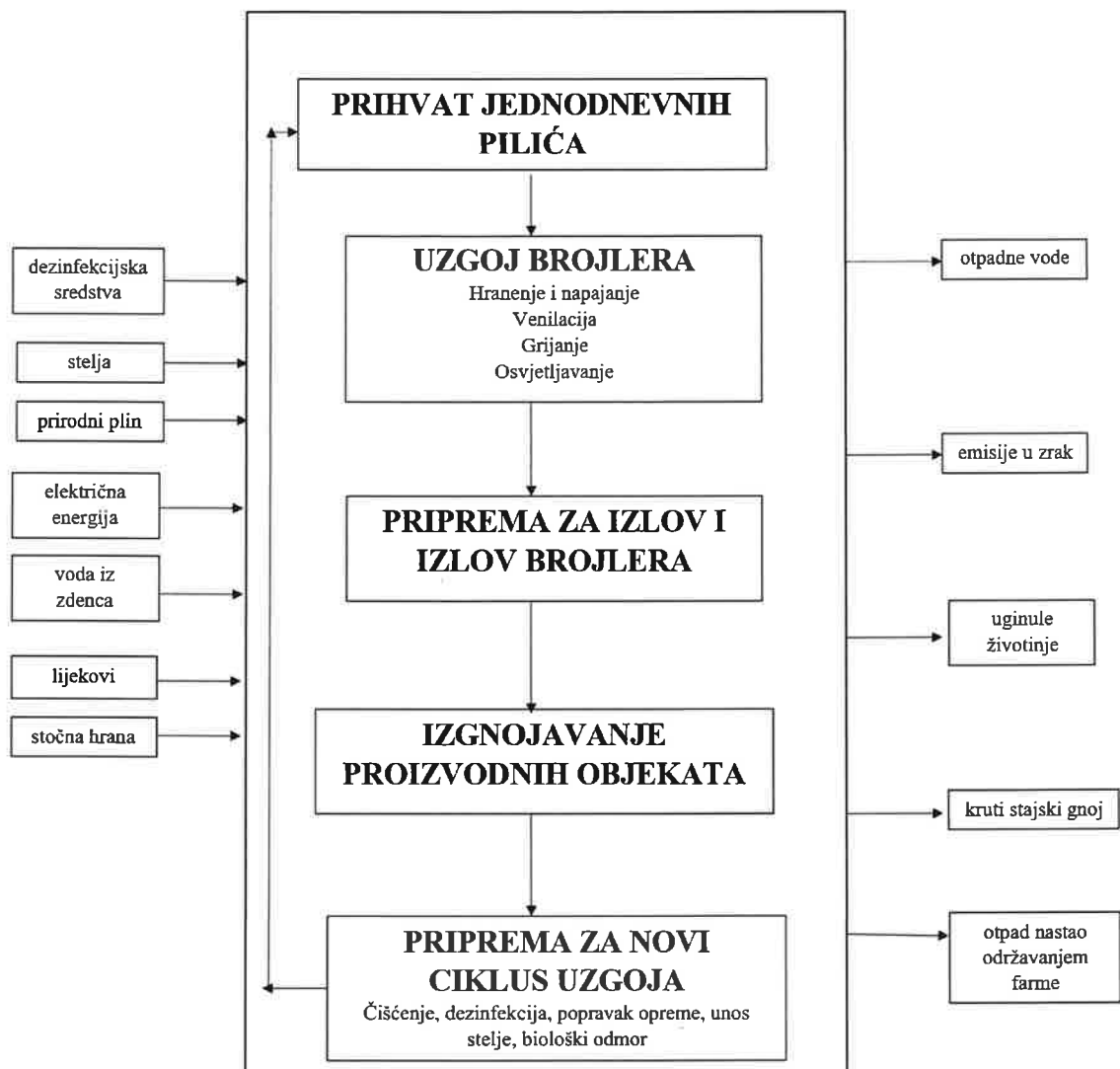
Prilog 2. Blok dijagram tehnološkog procesa na postojećem postrojenju za intenzivan uzgoj peradi Farma 13
